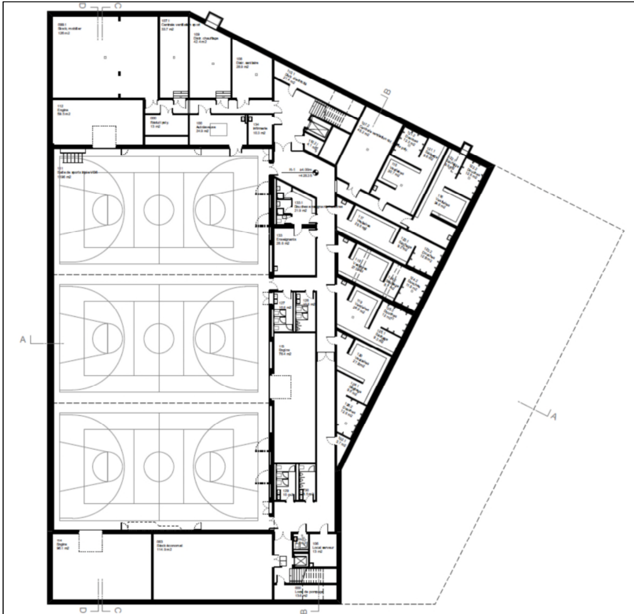
Collège : plan du sous-sol (salles sport)
