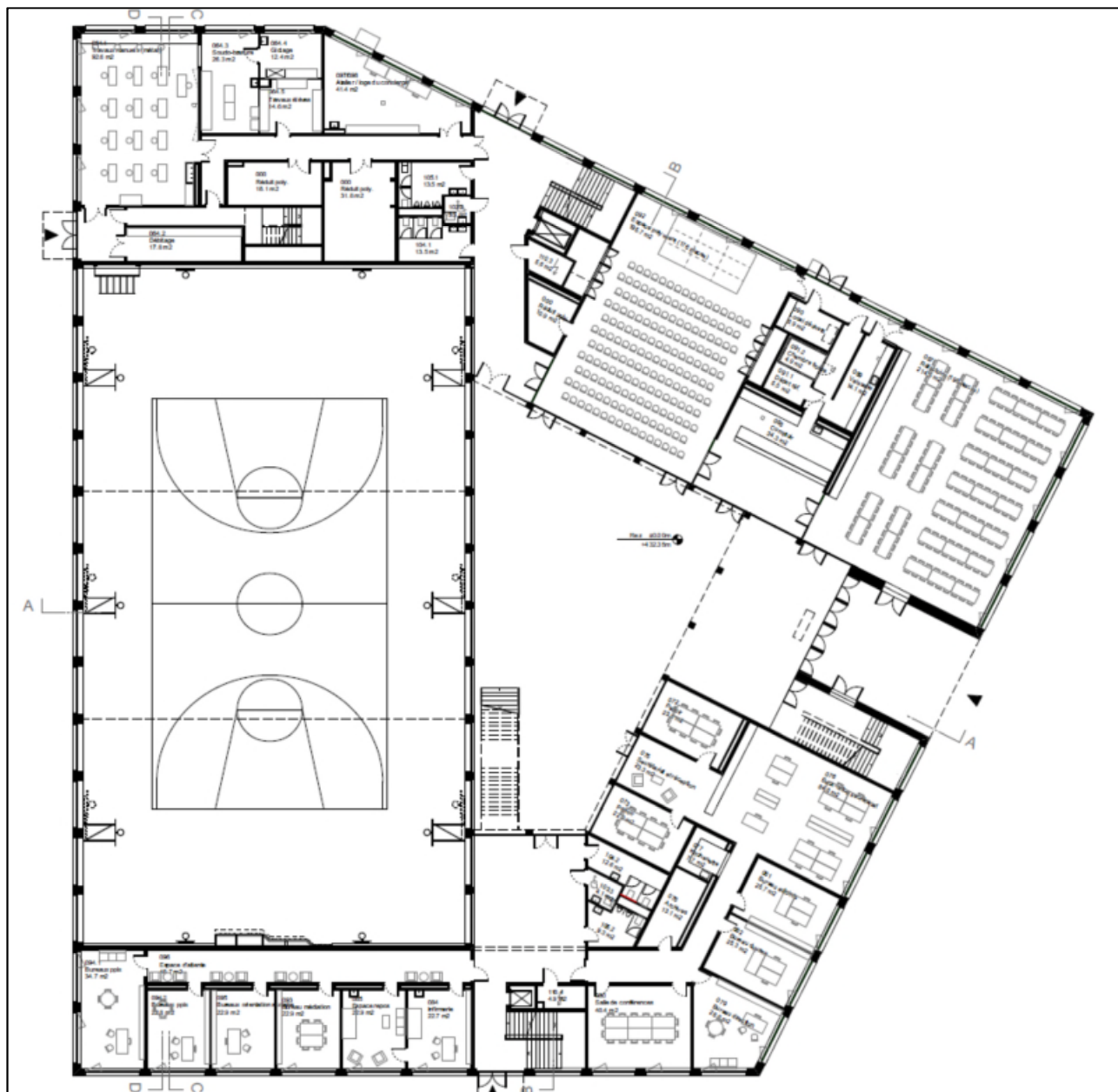
Collège : plan du rez-de-chaussée (entrée)
