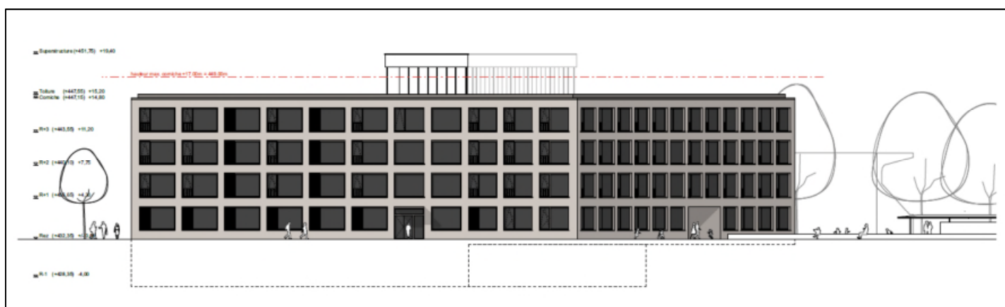
Collège : façade Sud
