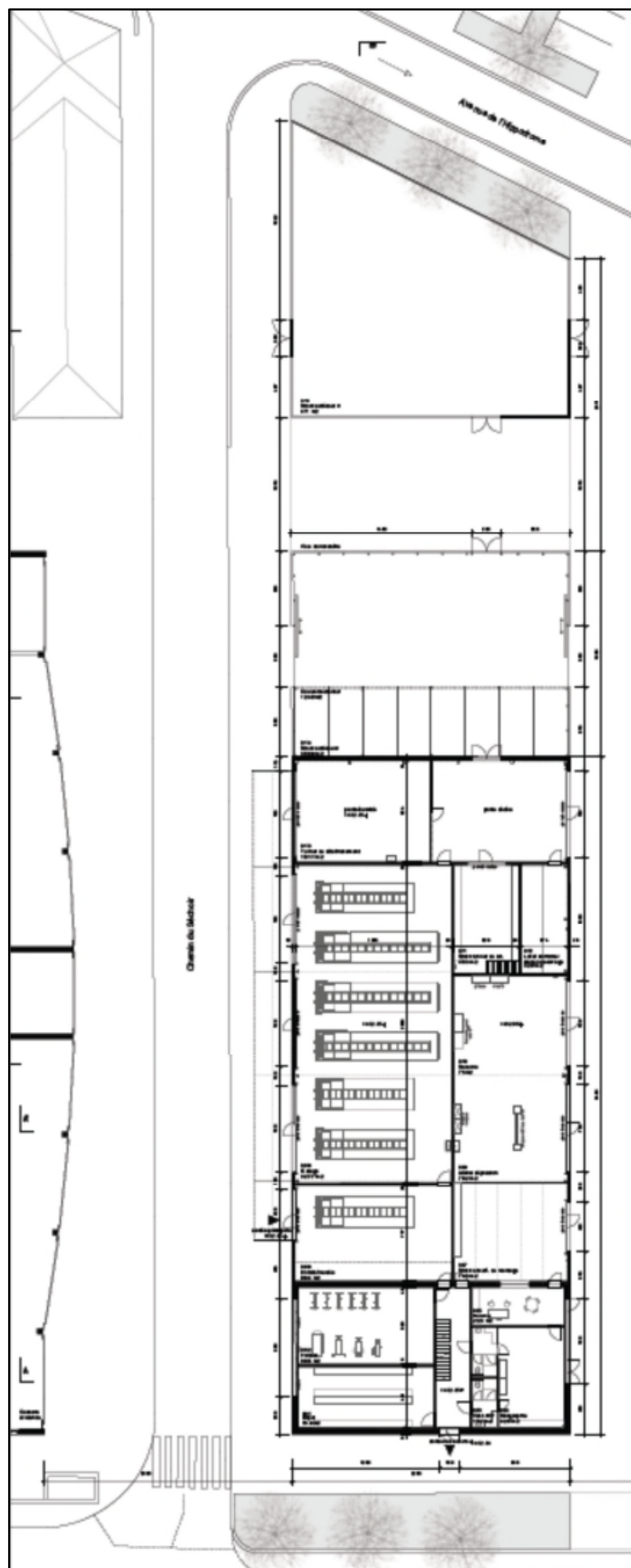
Extension de la caserne : plan du rez-de-chaussée
