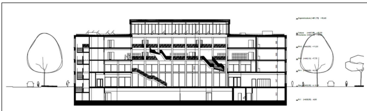
Collège : coupe Nord-Sud (sur l'atrium), en regardant l'Ouest
