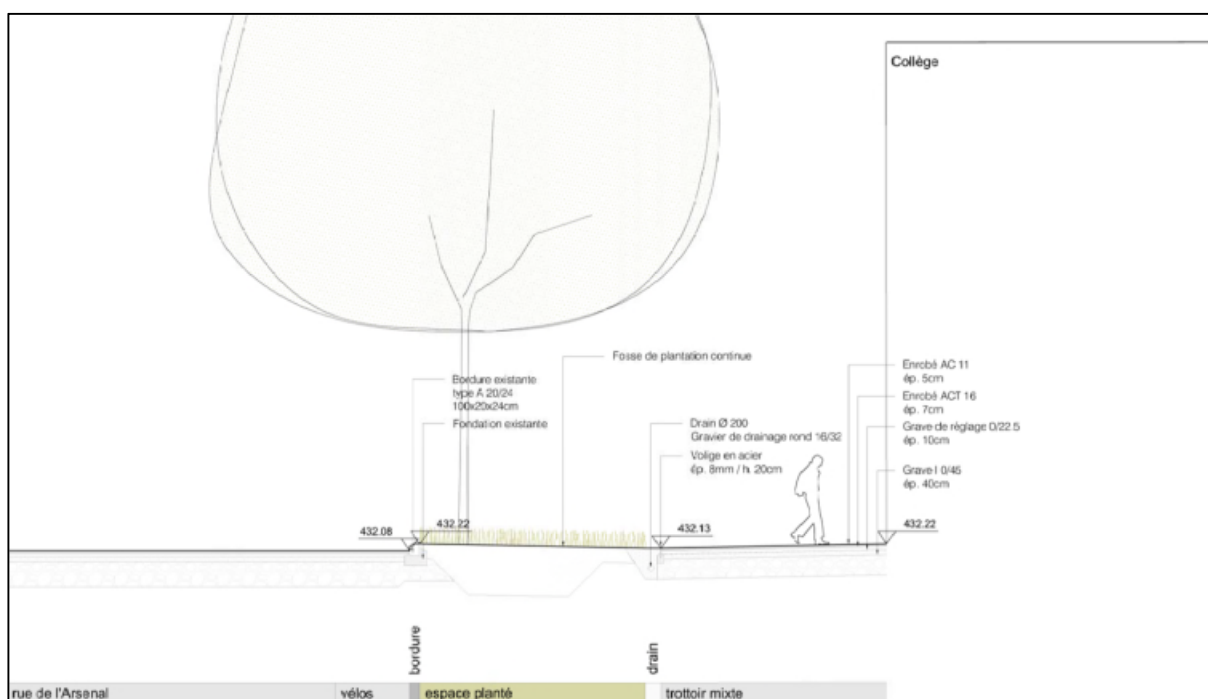
Rue de l'Arsenal : coupe sur le trottoir
