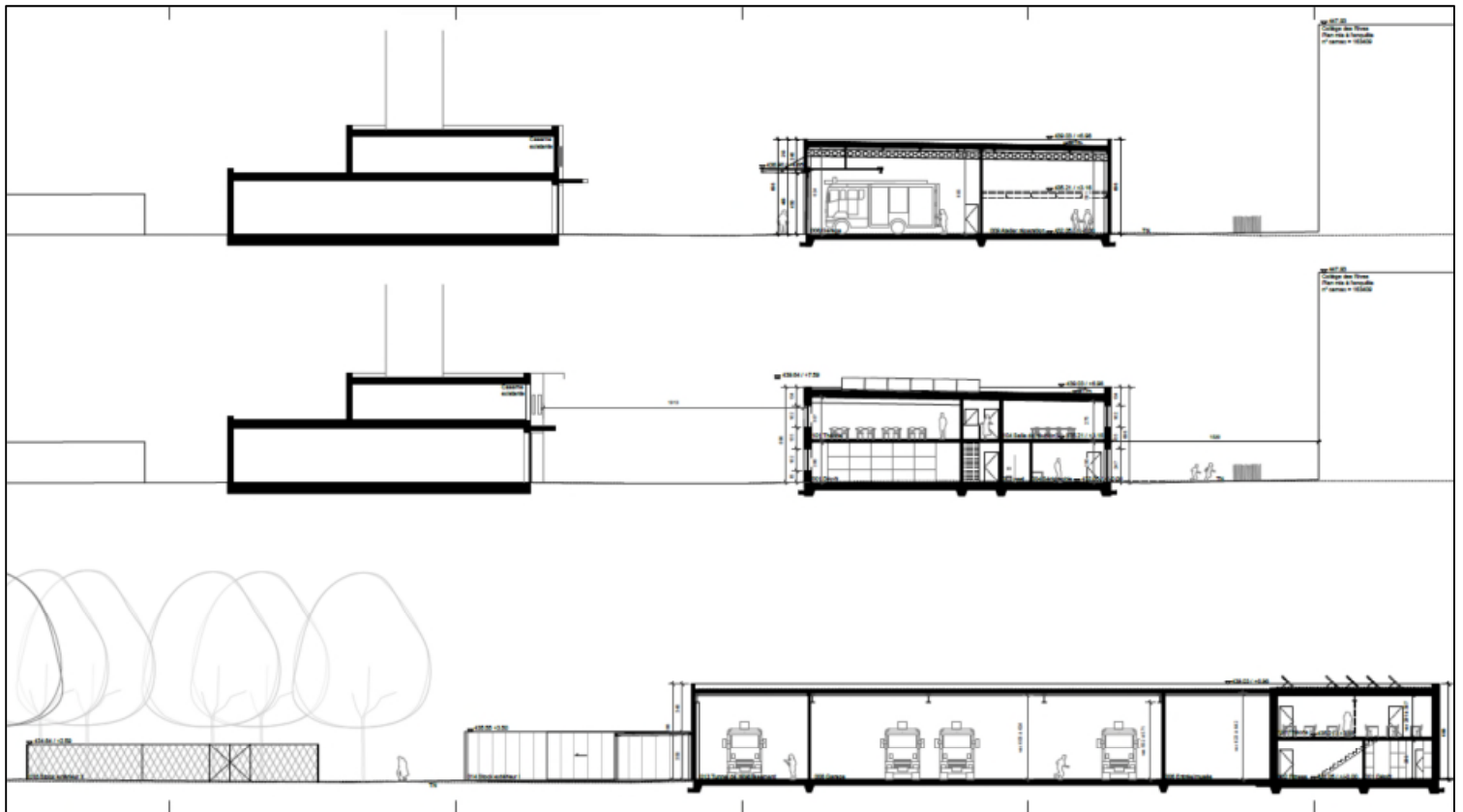
Extension de la caserne : coupes
