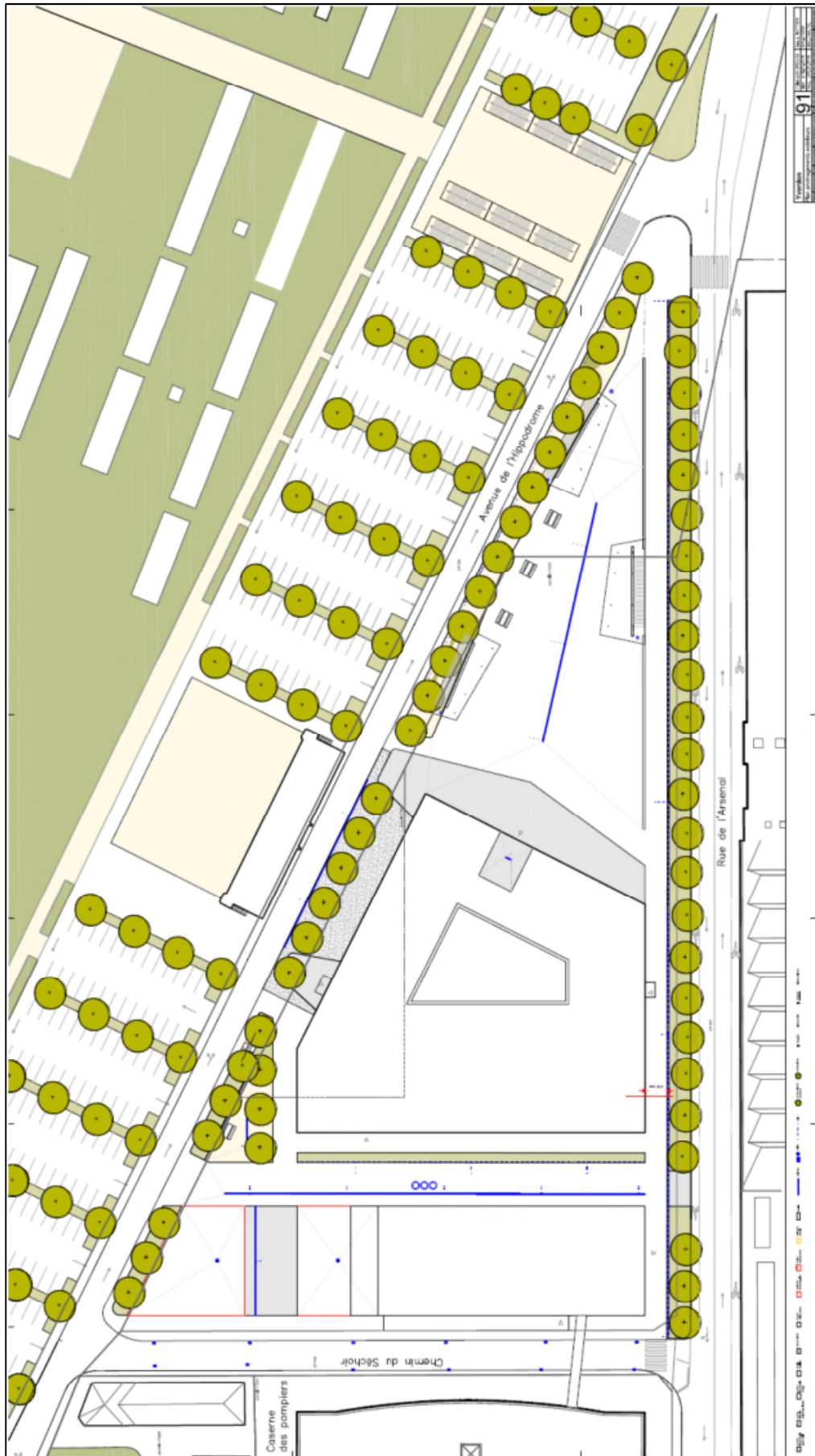
Collège et Caserne : vue générale, implantation et aménagements extérieurs
