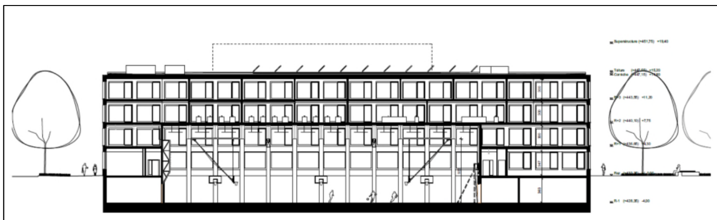
Collège : coupe Nord-Sud (sur la salle de gymnastique), en regardant l'Ouest
