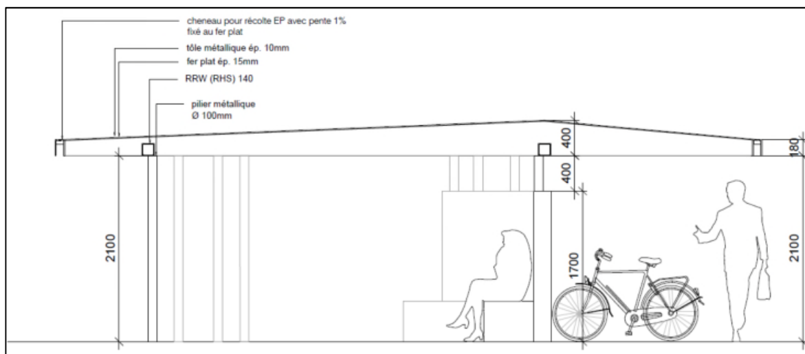
Stationnement Vélos 1 : coupe de principe, en lien avec les abris du préau
