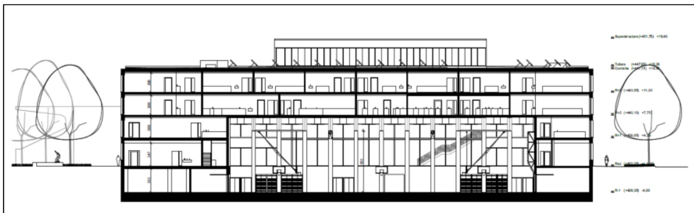
Collège : coupe Nord-Sud (sur la salle de gymnastique), en regardant l'Est
